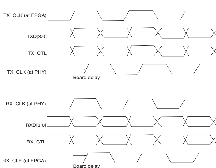
図2. RGMII のタイミング図
