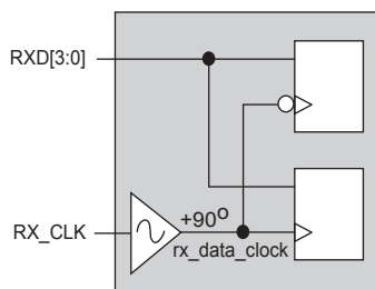
図 14. 遅延オプションをディセーブルした場合の RGMII 受信インタフェースの実装
