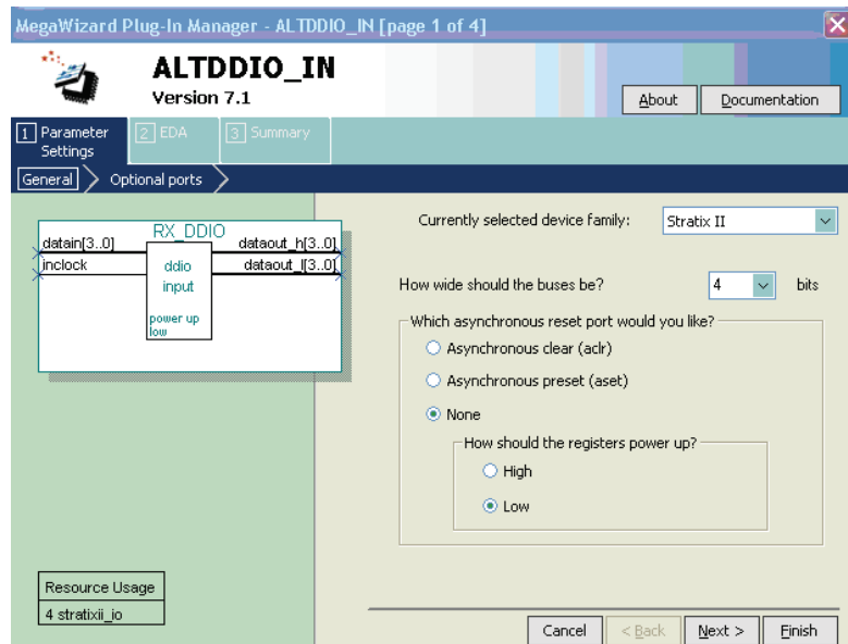
図 9. アルテラの受信インタフェース用 DDIO メガファンクション
