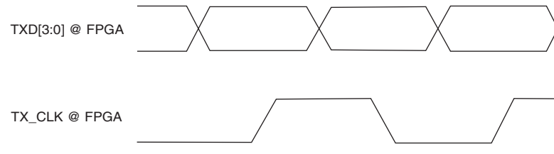
図 6. FPGA が生成する TX_CLK (PHY で TX_CLK 遅延をディセーブルした場合)
