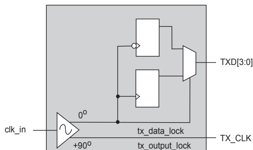
図 13. 遅延オプションをディセーブルした場合の RGMII 送信インタフェースの実装
