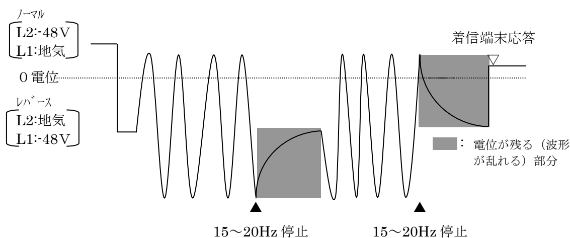
図 3.5.1 呼出信号送出時に印加される直流電圧（L1-L2 間）の例
