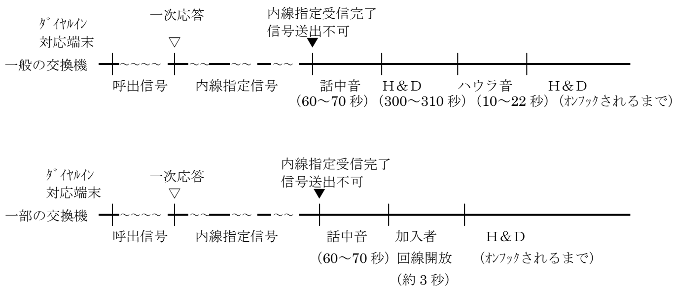
図 4.1.4 交換機のダイヤルインにおける切断シーケンス
