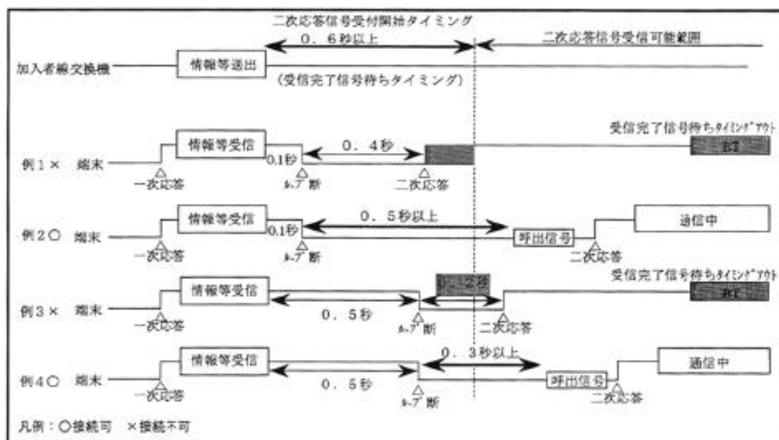
図 4.6.3 二次応答信号受付タイミングについて
