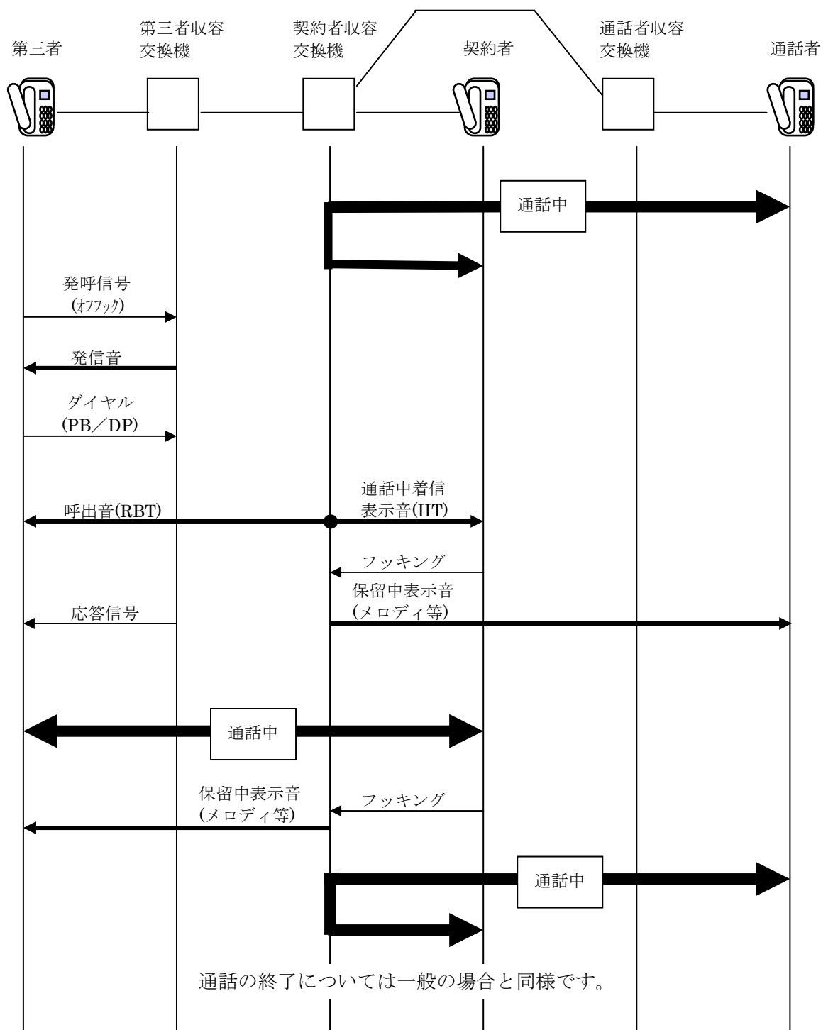
図 4.4.1 接続動作シーケンス例
