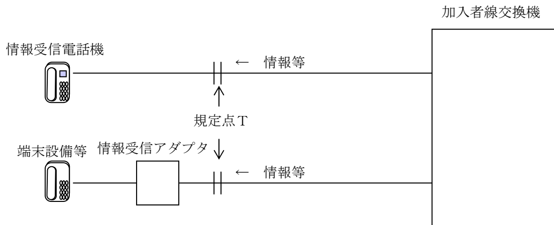
図 4.2.1 中継方式
