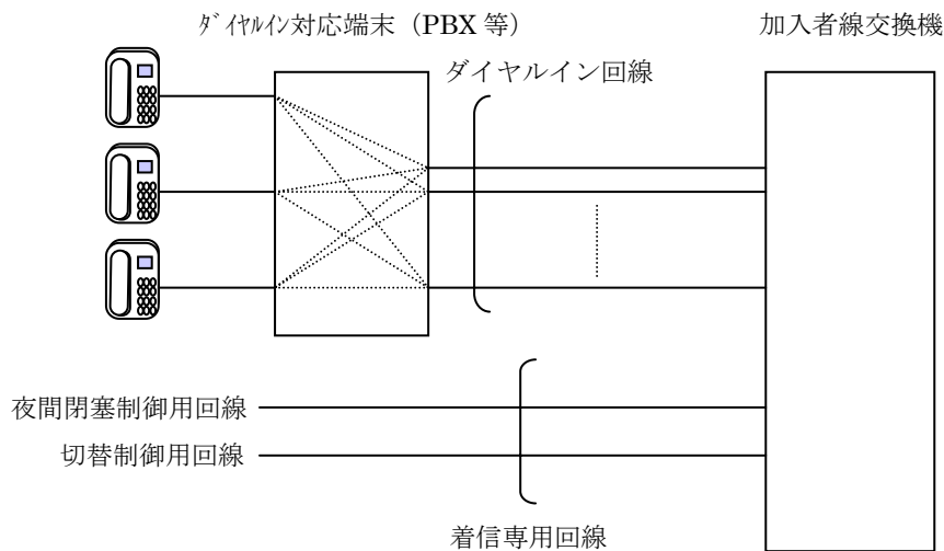
図 4.1.1 中継方式
