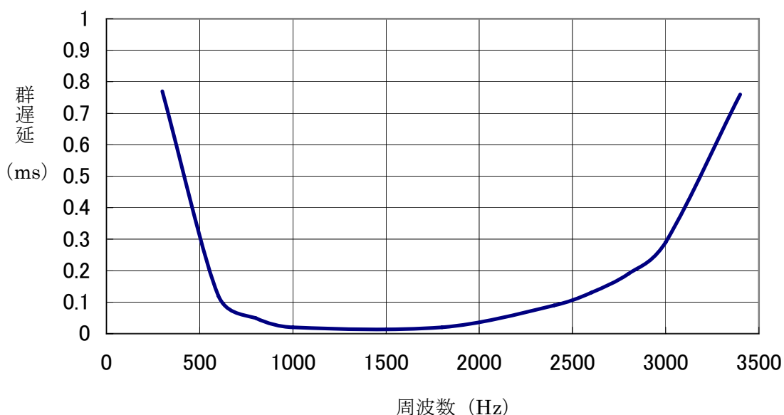
図 5.5.1 群遅延ひずみ
