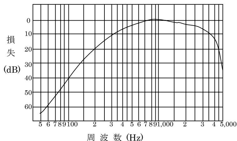
図 5.4.2 ITU-T 勧告の雑音評価特性
