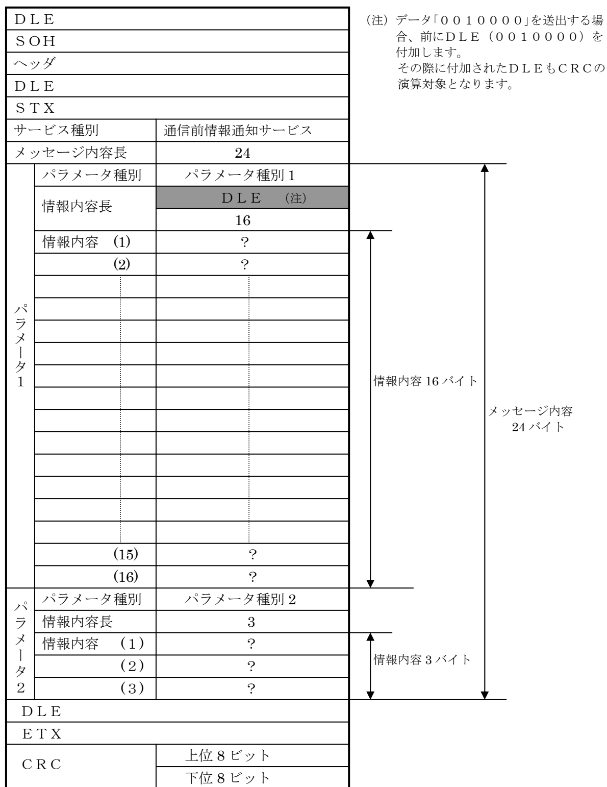
図 4.1.9 データフォーマットの留意事項
