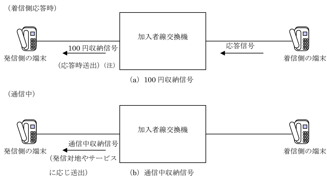
図 4.3.1 硬貨収納等信号送出時の接続状態【10 円単位課金の場合】
