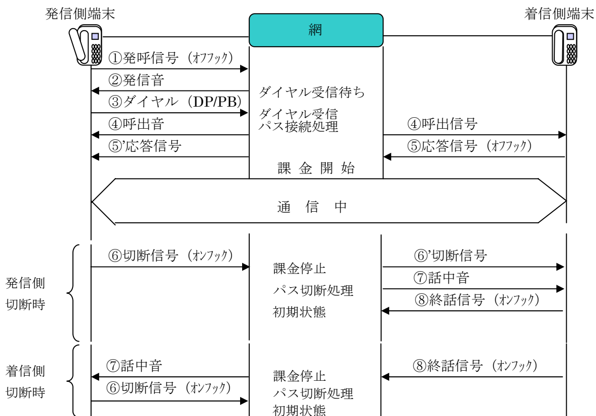
図 3.4.1 交換動作の概要
