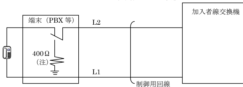
図 4.1.10 夜間閉塞時の接続処理
