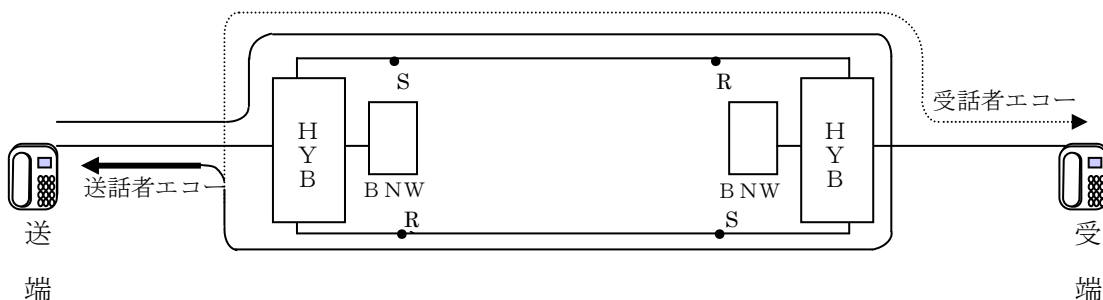
図 5.7.1 (4 線式－2 線式) 回線のエコー
