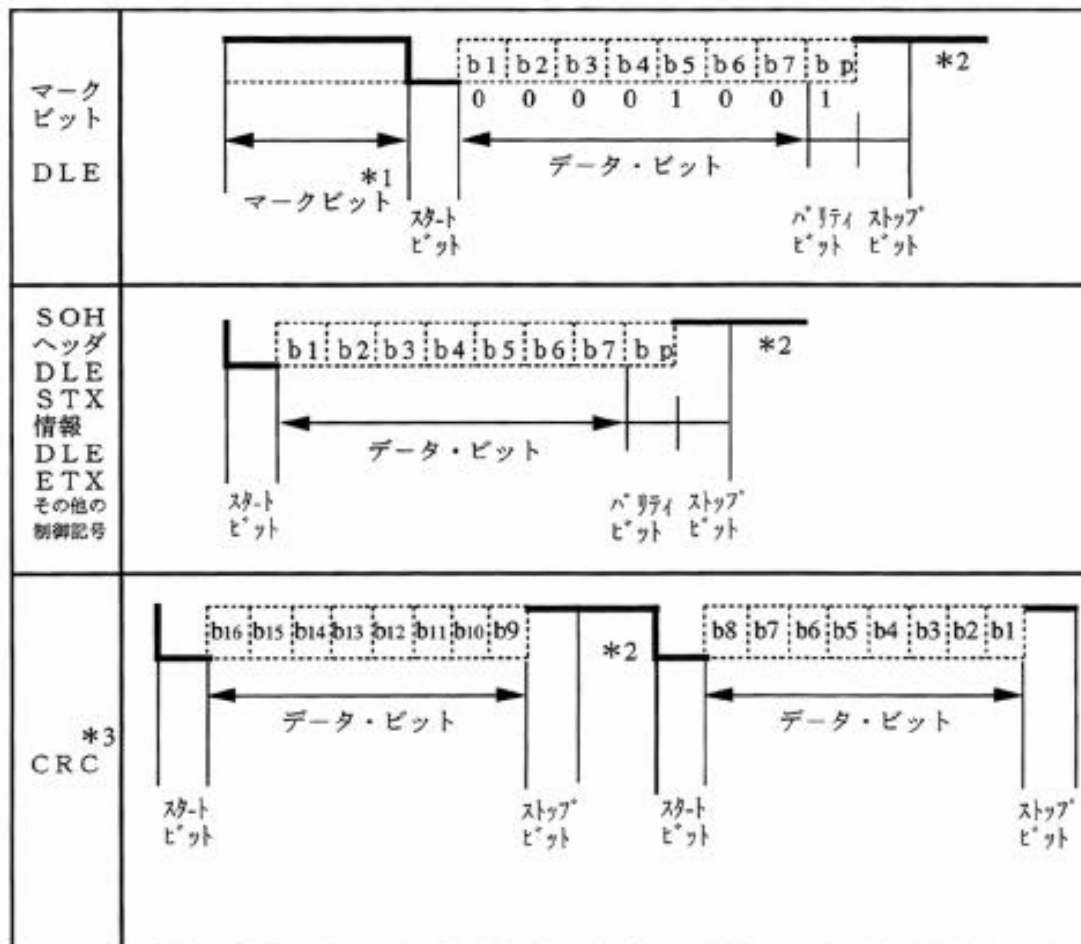
図 4.6.5 情報等の送出形式
