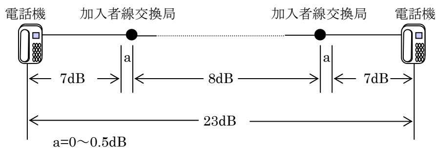
図 5.2.1 端末設備等相互間の回線の伝送損失
