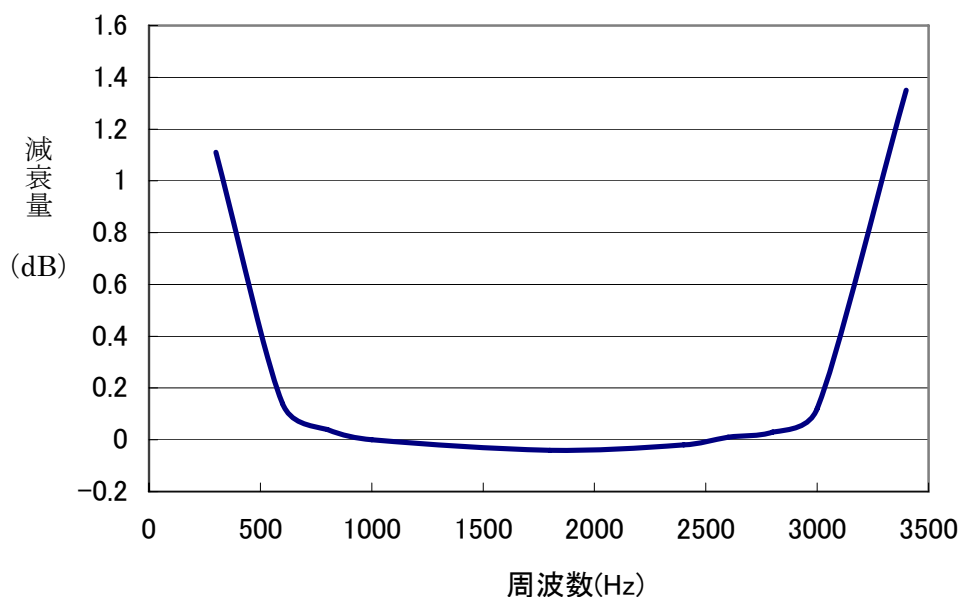
図 5.3.1 加入者線交換局－加入者線交換局間の減衰ひずみ
