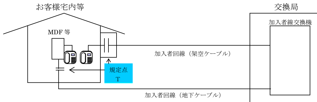
図 3.2.1 規定点
