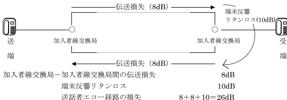
図 5.7.2 加入者線交換局—加入者線交換局間の送話者エコー経路の損失算出例
